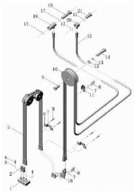
图 130/Fig.130 第三联附加油路(3 节门架)/3rd hydraulic vavle oil pipe(3-Stage mast)
