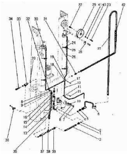
图 129/Fig.129 油路系统(3 节门架)/Mast piping (3-Stage mast)
