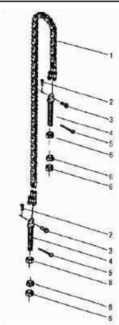
图 122/Fig.122 链条总成一(3 节门架)/Chain I (3-Stage mast)
