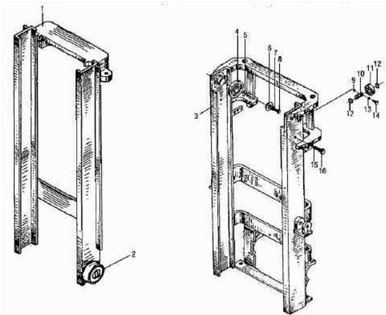
图 104/ Fig.104 门架(2 节门架)/Mast (Simplex)
