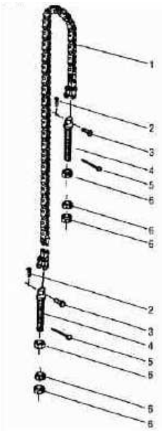
图 103/Fig.103 链条总成(2 节门架)/Chain (Simplex)
