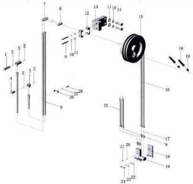
图 119/Fig.119 第四联附加油路(全自由、三节门架)/ 4th hydraulic vavle oil pipe （Full free & 3-Stage mast）
