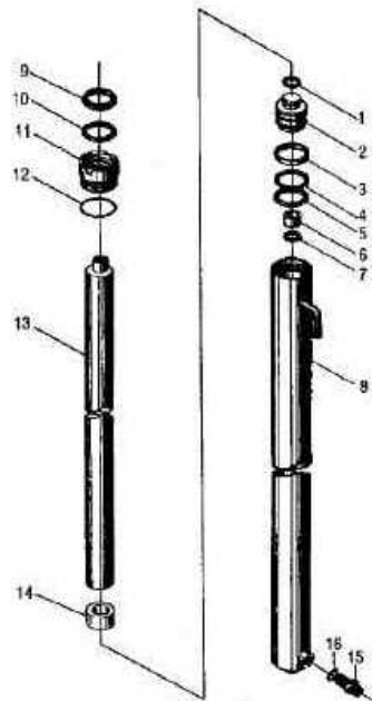
图 106/ Fig.106 左、右升降油缸(2 节门架)Lifting cylinder, Left & Right (Simplex)
