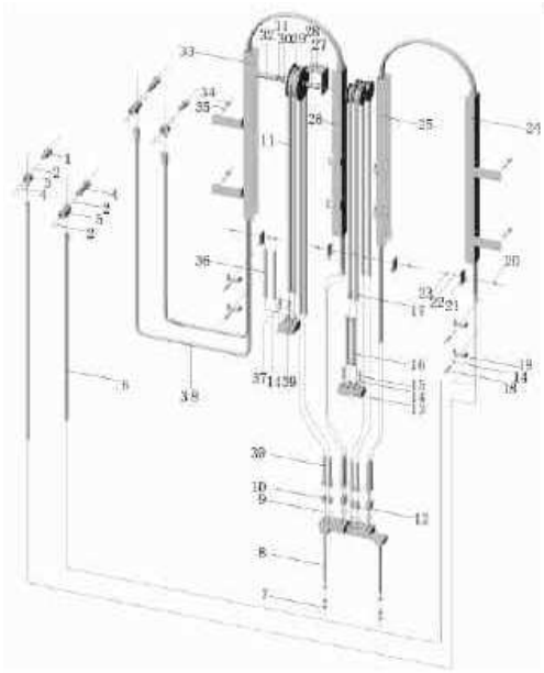
图 120/Fig.120 第三、四联附加油路(全自由门架)/ 3rd & 4th hydraulic vavle oil pipe （Full free mast）
