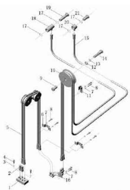
图 130/ Fig.130 第三联附加油路(3 节门架)/3rd hydraulic vavle oil pipe(3-Stage mast)
