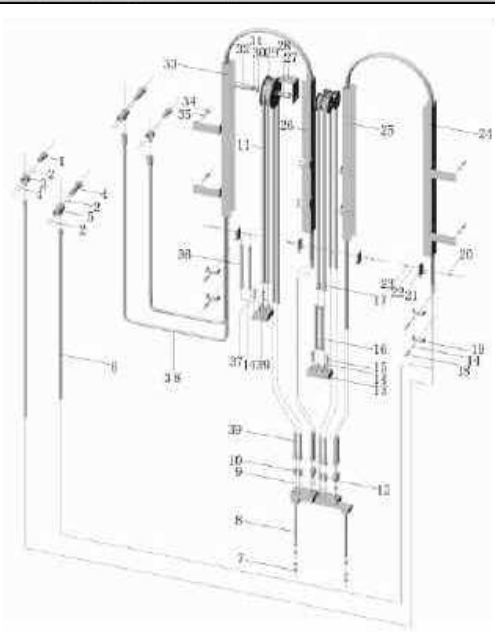
图 120/Fig.120 第三、四联附加油路(全自由门架)/ 3rd & 4th hydraulic vavle oil pipe （Full free mast）
