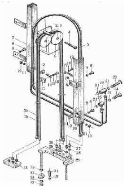
图 118/Fig.118 第三联附加油路(2 节全自由门架)/3rd hydraulic vavle oil pipe（Free lift mast）
