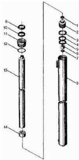
图 127-1/Fig.127-1 左、右升降油缸(3 节门架)/Lift cylinder,left & right (3-Stage mast)
