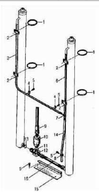
图 108/Fig.108 油路系统(2 节门架)/Oil pipe system(Simplex)
