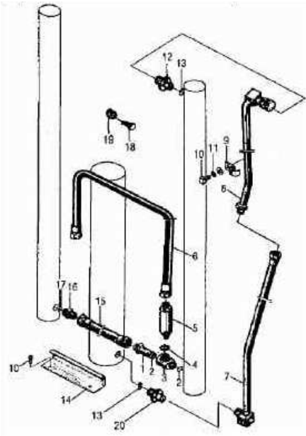
图 117/Fig.117 油路系统(2 节全自由门架)/Mast piping (Free lift mast)
