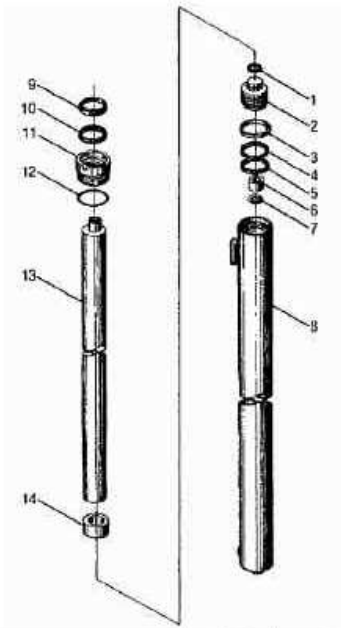
图 127-1/Fig.127-1 左、右升降油缸(3 节门架)/Lift cylinder,left & right (3-Stage mast)
