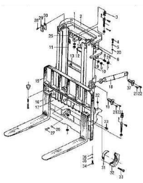
图 102/Fig.102 起升组件(2 节门架)/Lifting part (Simplex)
